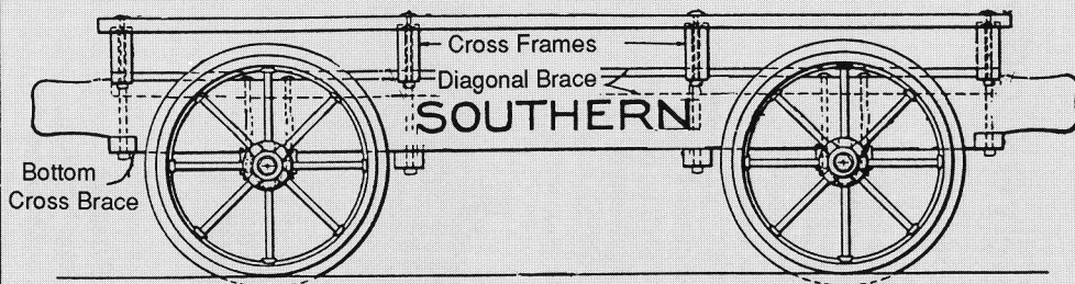
Elevation
